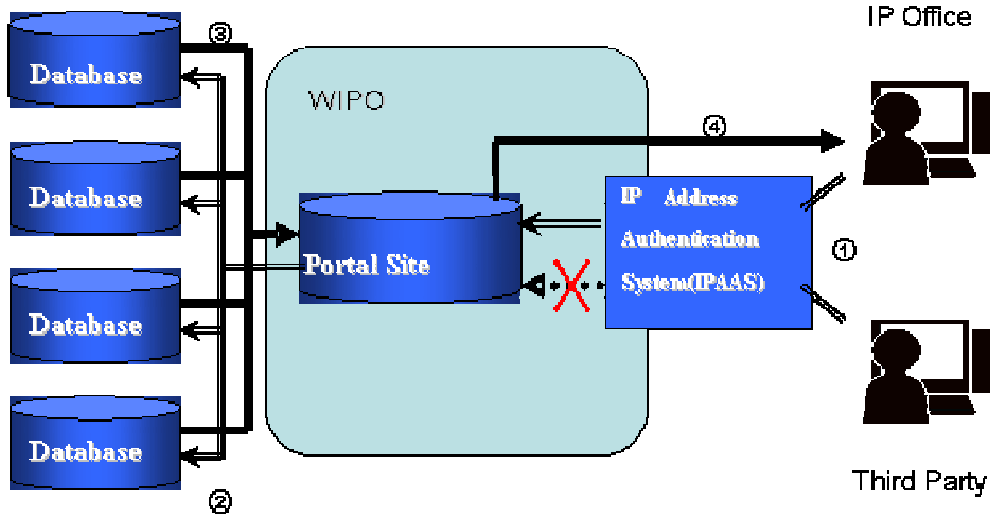
Рисунок 1: Общий вид комплексной системы поиска баз данных для индивидуальных баз данных государств-членов ВОИС
